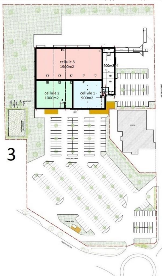
Exemples de schémas de découpage du bâtiment en cellules d'activité
